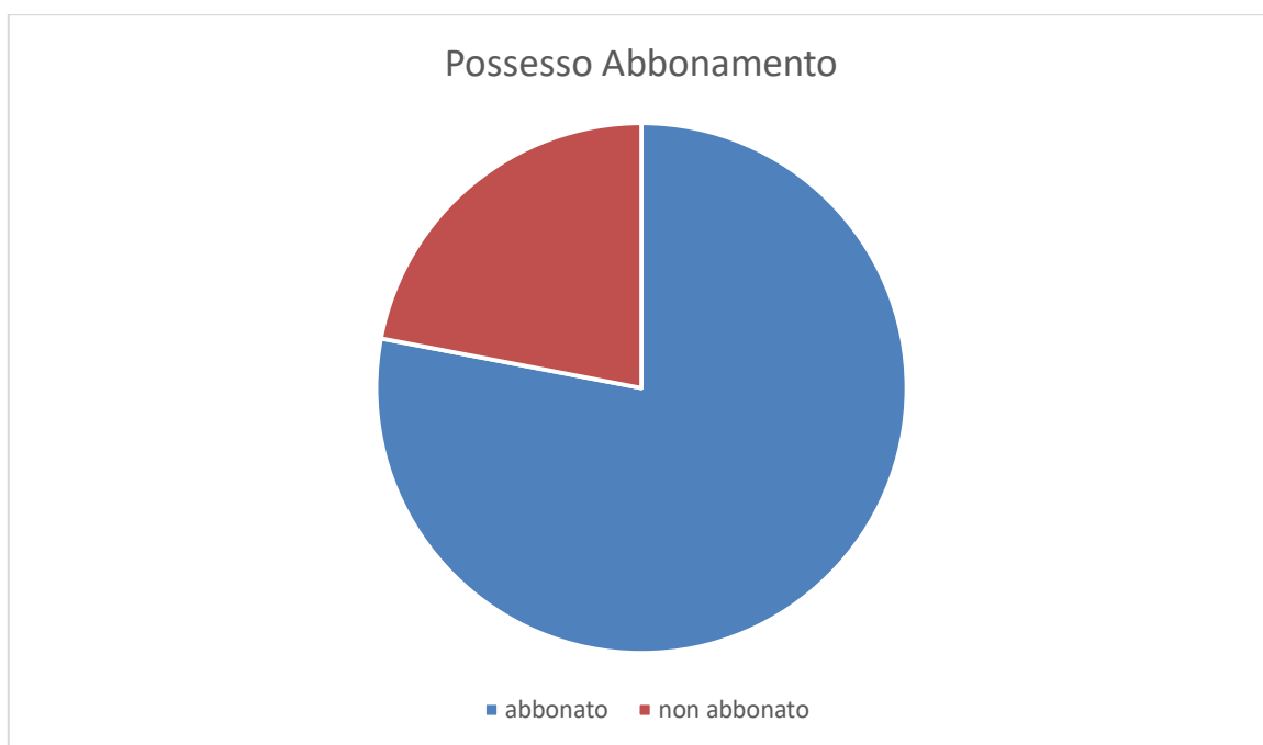
Grafico.3 Possesso abbonamento
